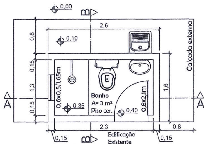
PLANTA BAIXA A= 4,16 m²
